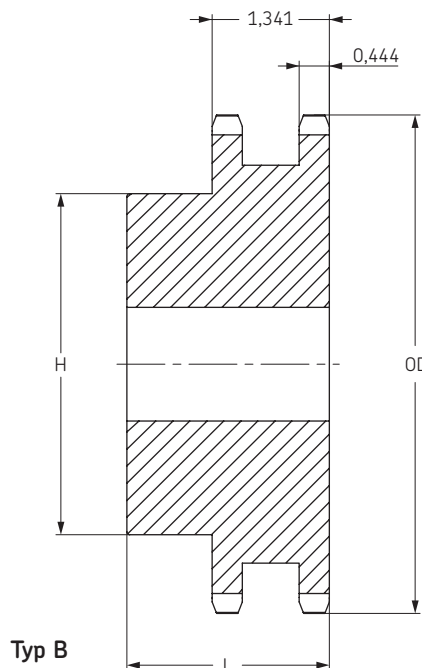
S předvrtanou dírou Typ B
