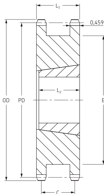
Typ A Kuželové pouzdro
