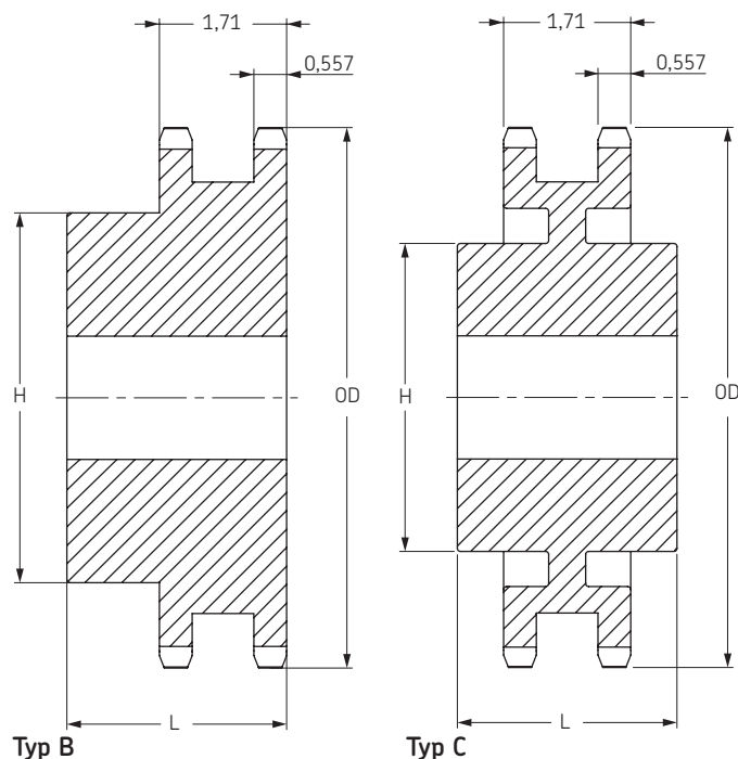
S předvrtanou dírou Typ B
