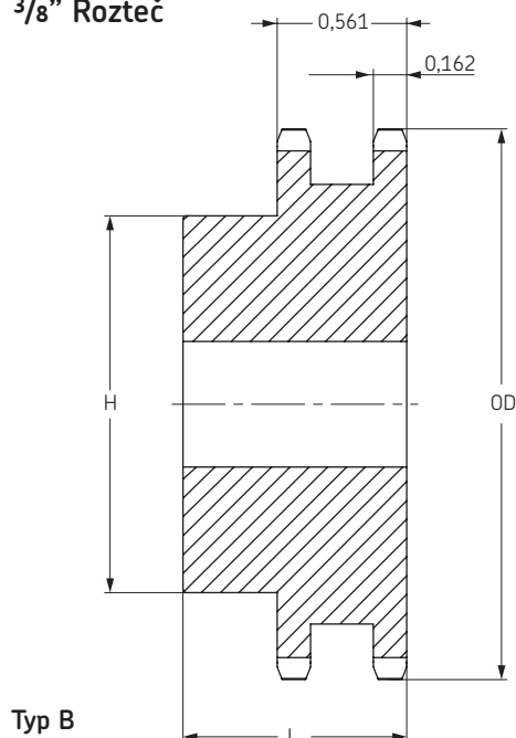
ANSI 35-2 3/8" Rozteč
