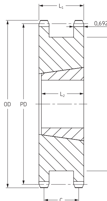
Typ A Kuželové pouzdro
