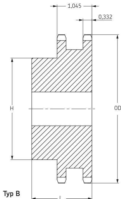
S předvrtanou dírou Typ B
