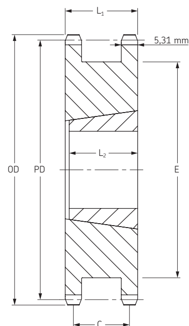
Typ A Kuželové Pouzdro
