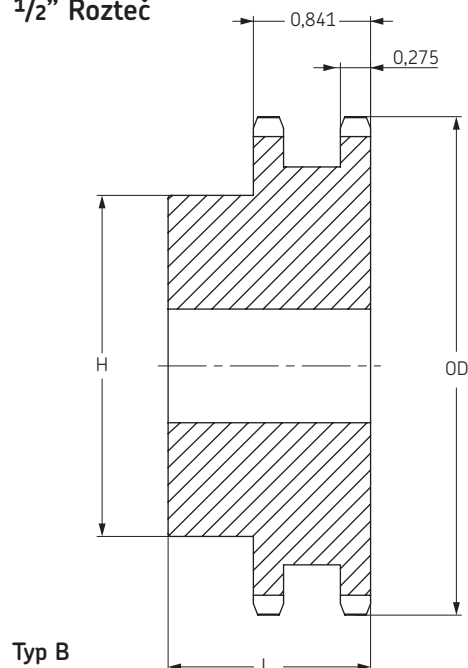
ANSI 40-2 1/2" Rozteč
